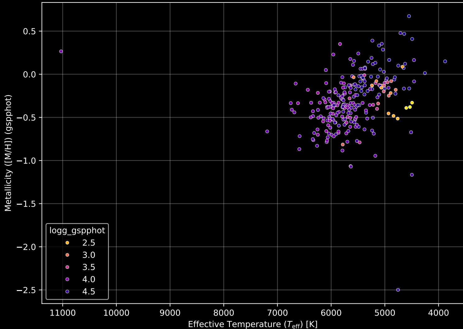
GALAH DR4 Field: [521] Stellar Population Parameters (n= 259)
