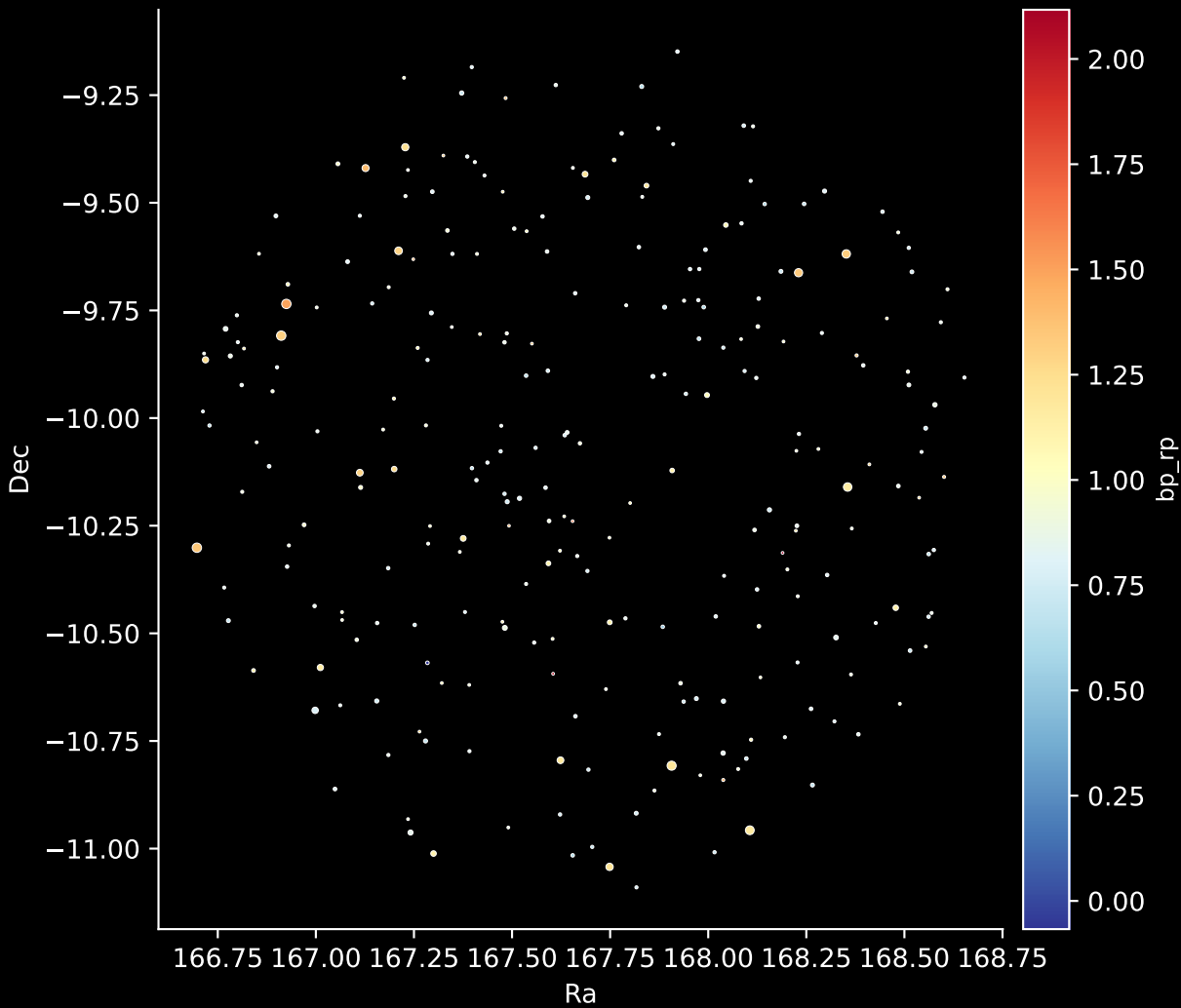
GALAH DR4 Field: [521] Stars: 259
